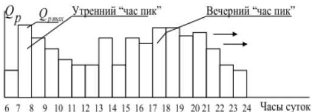
Рисунок 3 - Эпюра расчётных величин пассажиропотока по часам суток
