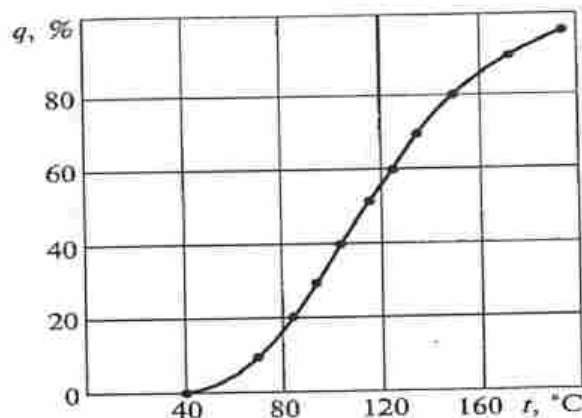
Рисунок 1 – Кривая перегонки бензина:
